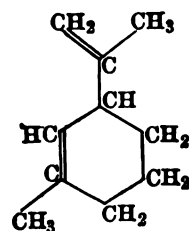
Sylvestrene.
